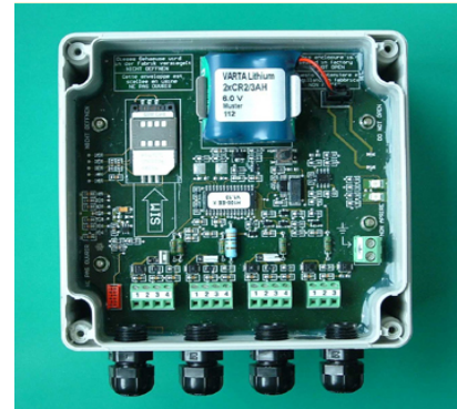
Sendegerät
